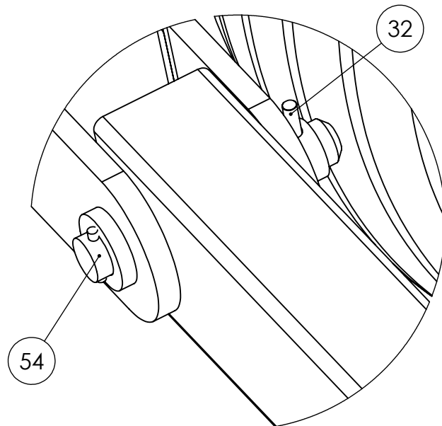
32 54 DETAIL R 1:4
