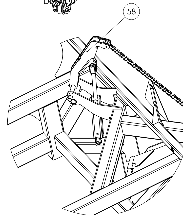
58 DETAIL Y 1:16
